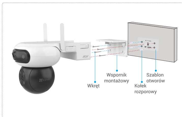
Rys. 2 Montaż ścienny
