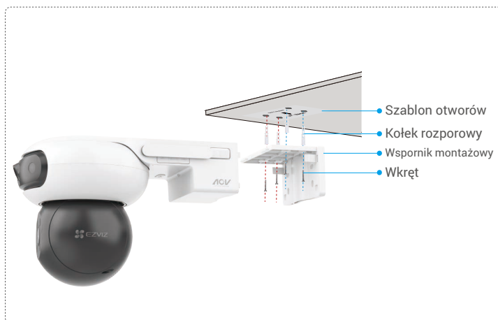
Rys. 1 Montaż sufitowy
